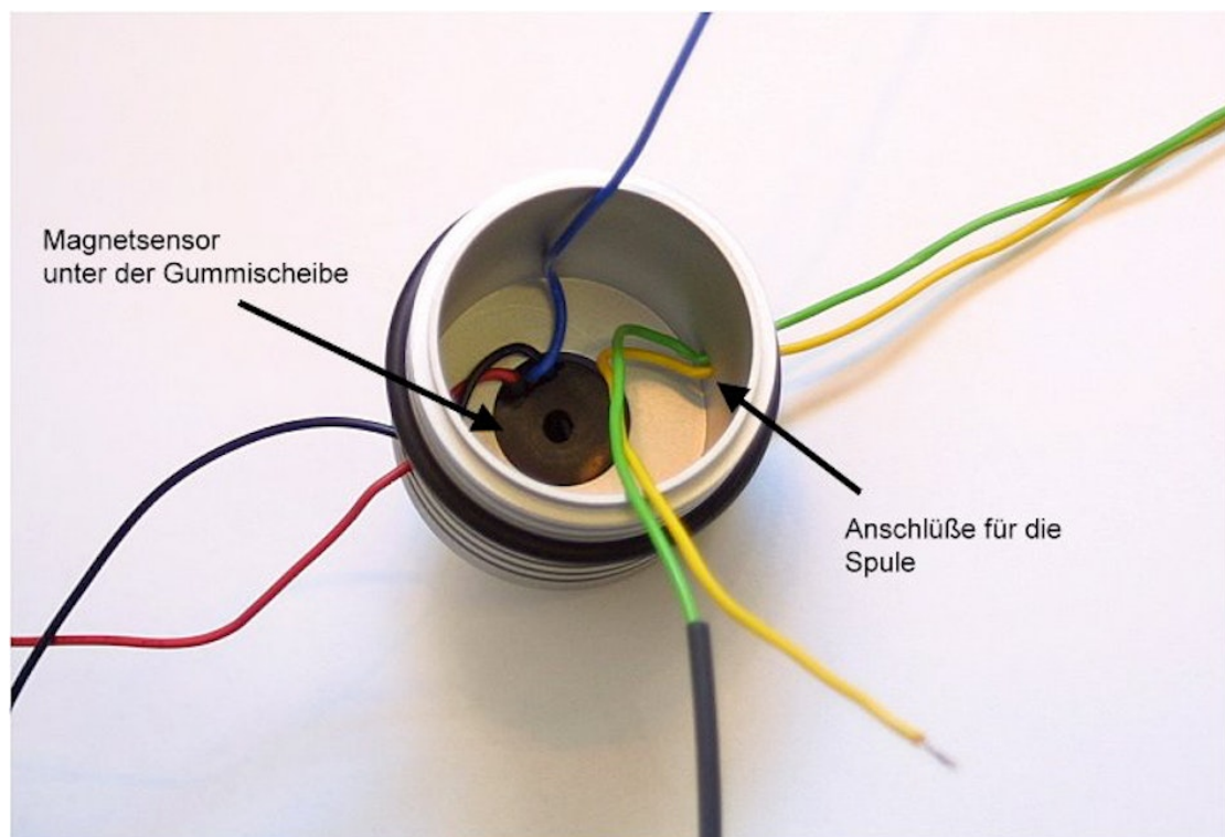
Sguardo all'interno del supporto: il sensore a effetto Hall viene fissato alla punta del supporto con un disco di gomma.
