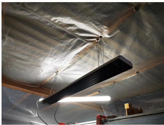
Fixation au plafond du radiateur à infrarouge relativement lourd : 4 OTN-40 - aimants en pot avec œillet ( www.supermagnete.it/fre/OTN-40 )
